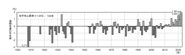
図表 2-1-4 釧路沖の海域平均海面水温(年平均)の偏差の推移 (1908年~2022年)
